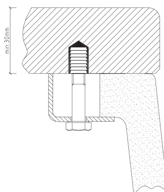
Montážní schema
