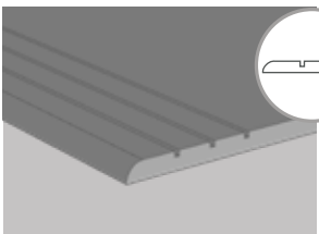
LAV. MONOLITE “MONOLITE” SHAPE Volume aperto per l’istallazione di tasselli a scomparsa. Volume aperto per l’istallazione di tasselli a scomparsa.
