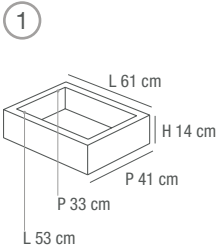
LAVABO DAVE DA APPOGGIO LAVORAZIONE A “DOPPIA L” CON VASCA L (33x53 cm) LEANING DAVE WASHBASIN “DOUBLE L” SHAPE CON SINK L (33x53 cm)
