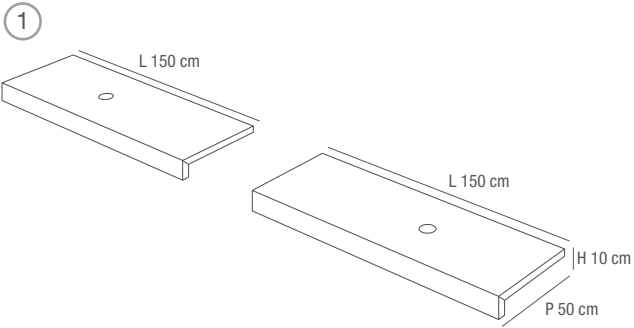
TOP LAVORAZIONE A “L” TOP “L” SHAPE
