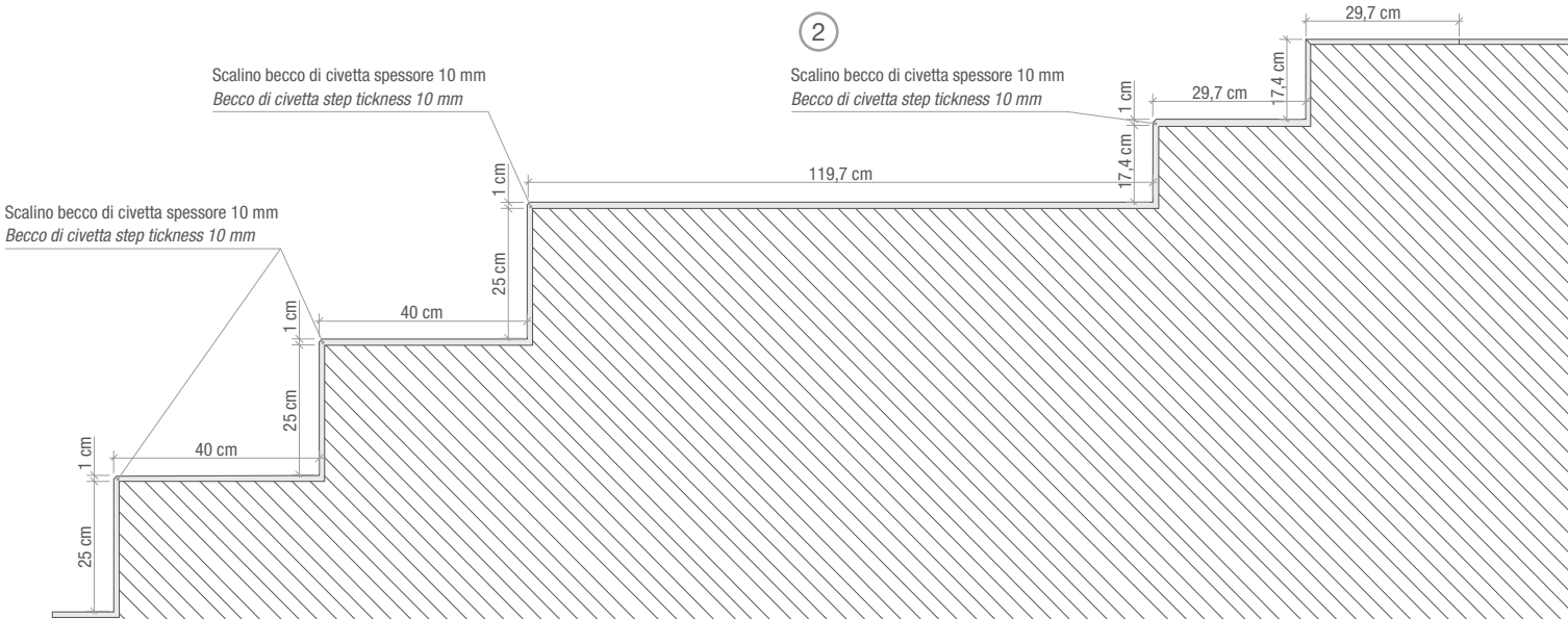
SCALINI LAVORAZIONE A “BECCO DI CIVETTA” STEPS LAVORAZIONE A “BECCO DI CIVETTA”
