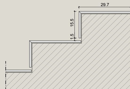
Sezione scalini
